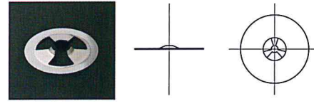
<三ツ爪 スピードワッシャ>
